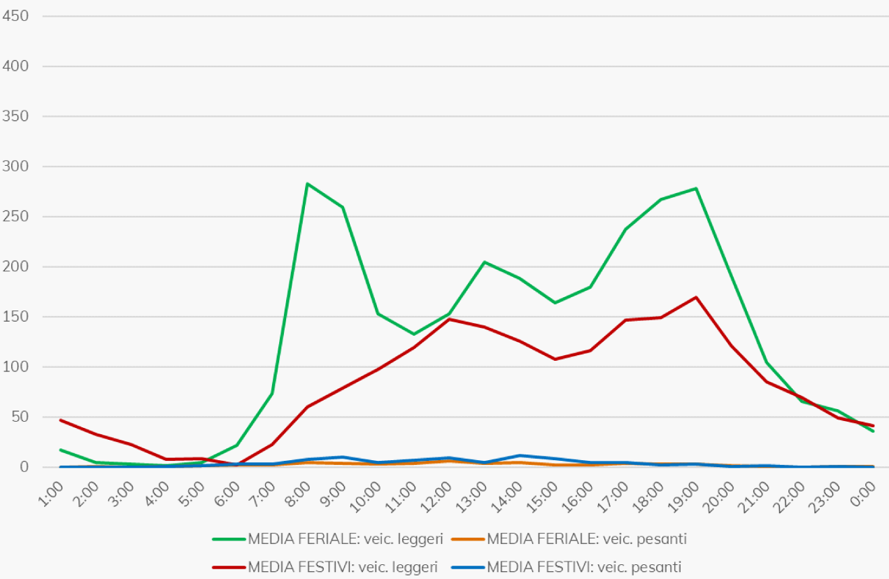
FLUSSO (accorpamento orario) direzione NORD 17/01/2023 - 23/01/2023
