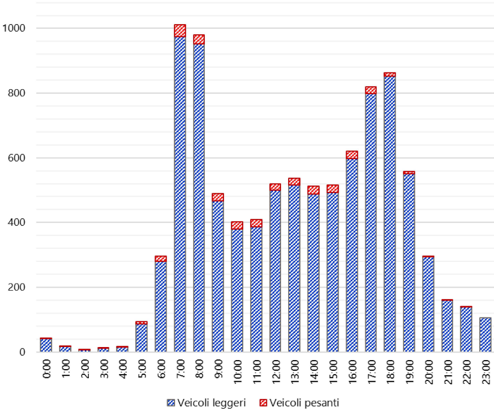
ANDAMENTO GIORNALIERO MEDIO DEI FLUSSI BIDIREZIONALI
