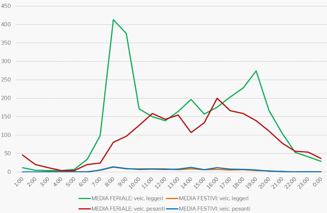
FLUSSO (accorpamento orario) direzione SUD 17/01/2023 - 23/01/2023
